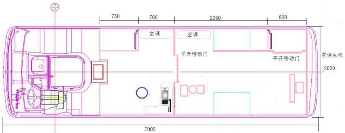
(检查区设计布局图)
